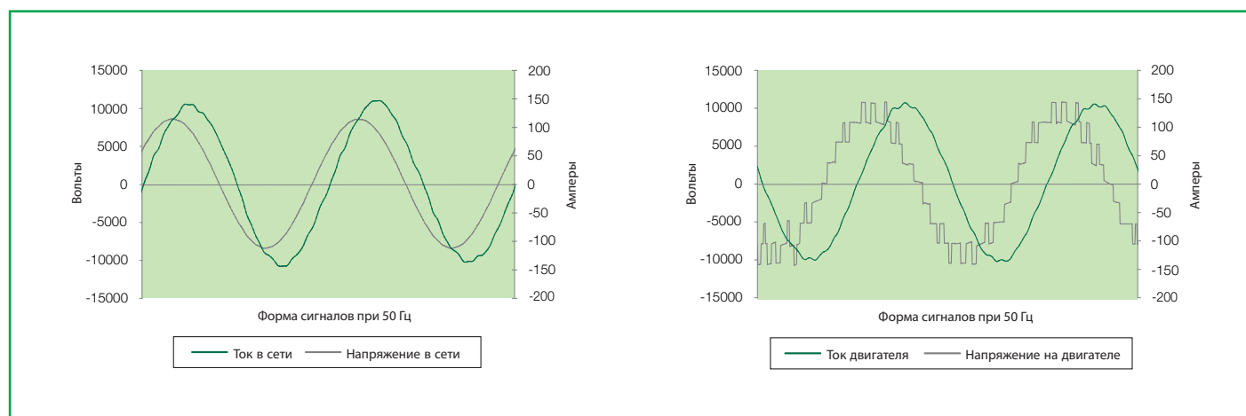
Ток и напряжение электродвигателя и питающей сети
