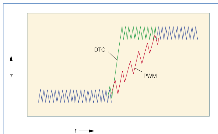
Типичная характеристика крутящего момента (Т) привода с прямым управлением моментом в сравнении с векторным управлением
