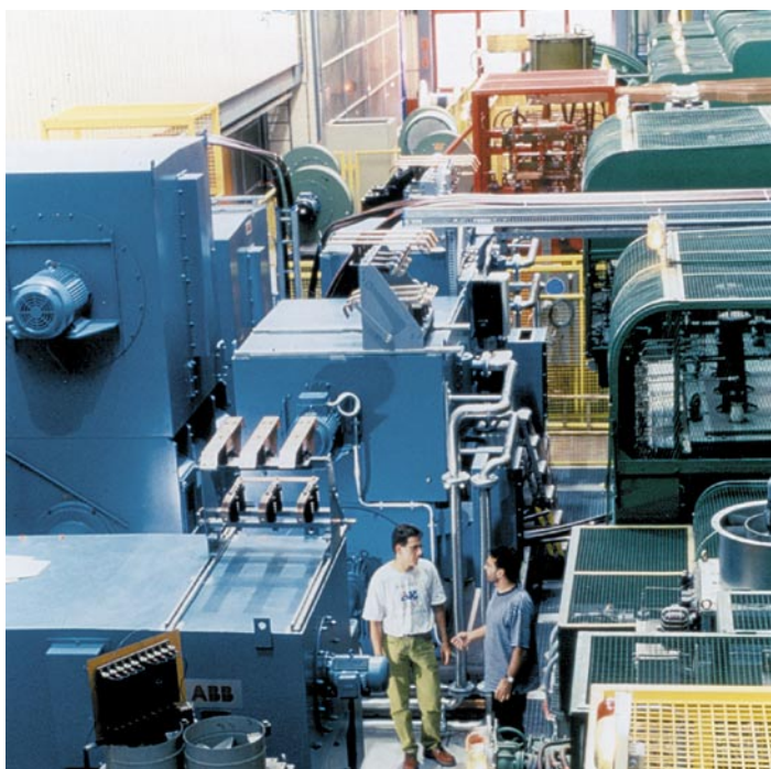
Испытательное оборудование ABB на заводе - изготовителе приводов в Швейцарии. Прежде чем привод будет отгружен заказчику, каждый привод ACS 1000 подвергается испытаниям под нагрузкой, управляя нагруженным двигателем среднего напряжения,
